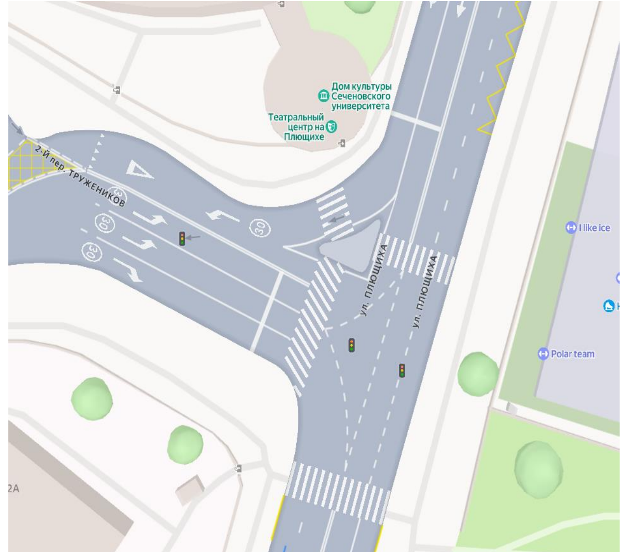
Ситуационный план
